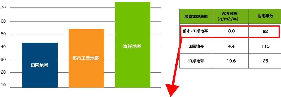
亜鉛付着量と環境別耐用年数の関係
