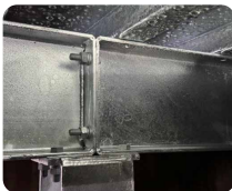
支柱と梁
